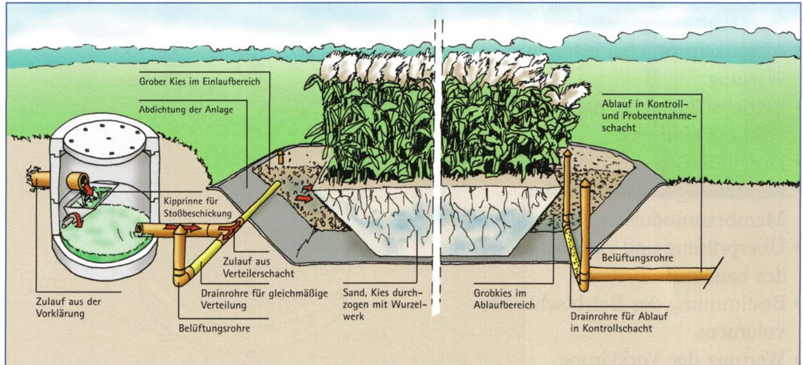
Abb. 21 Horizontal durchflossene Pflanzenstufe
