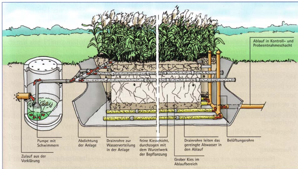
Abb. 23 Vertikal durchflossene Pflanzenanlage
